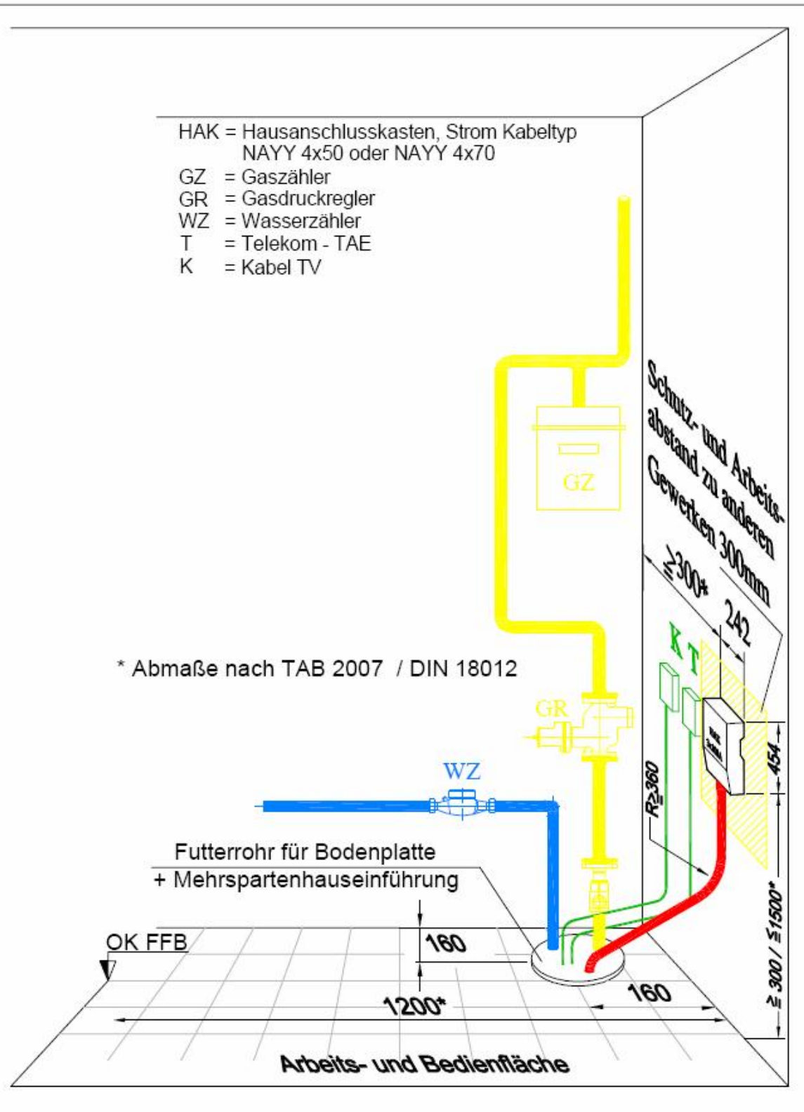
Abbildung 2: Installationsvariante Mehrspartenhausanschluss, vertikaler Einbau für nicht unterkellerte Gebäude
